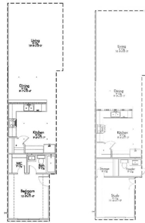
1.) BEDROOM SUITE
